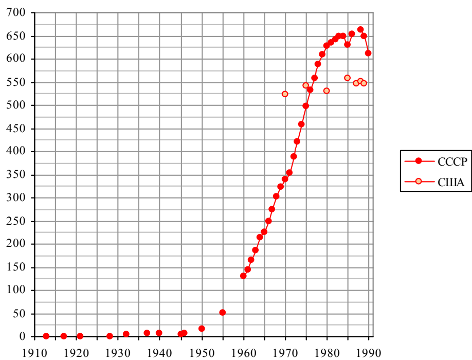
Перекачка нефти и нефтепродуктов по нефте- и нефтепродуктопроводам, млн. тонн. Источники: [3, S.3, S.21].
