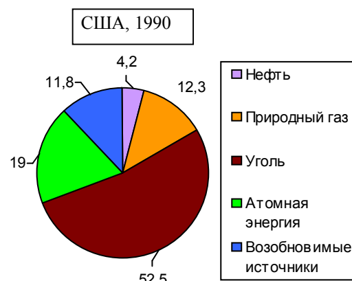
Производство электроэнергии, млрд. кВт*ч. Источники: [1, 3, 12, 13, 14, 28, 57, S.3, S.6, S.12, S.14, S.15, S.17, S.18, S.19, S.46, S.63, S.67].
