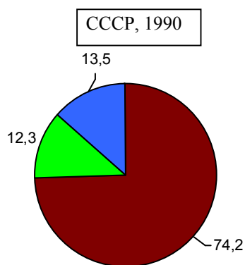
Производство электроэнергии, млрд. кВт*ч. Источники: [1, 3, 12, 13, 14, 28, 57, S.3, S.6, S.12, S.14, S.15, S.17, S.18, S.19, S.46, S.63, S.67].
