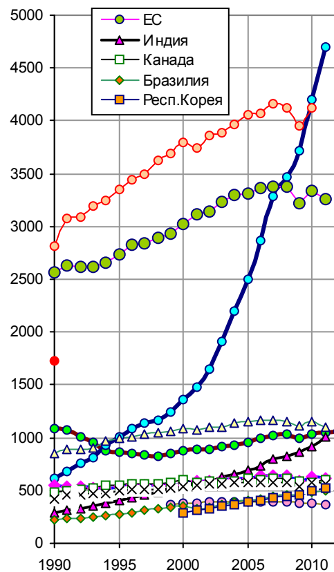
Производство электроэнергии, млрд. кВт*ч. Источники: [1, 3, 12, 13, 14, 28, 57, S.3, S.6, S.12, S.14, S.15, S.17, S.18, S.19, S.46, S.63, S.67].
