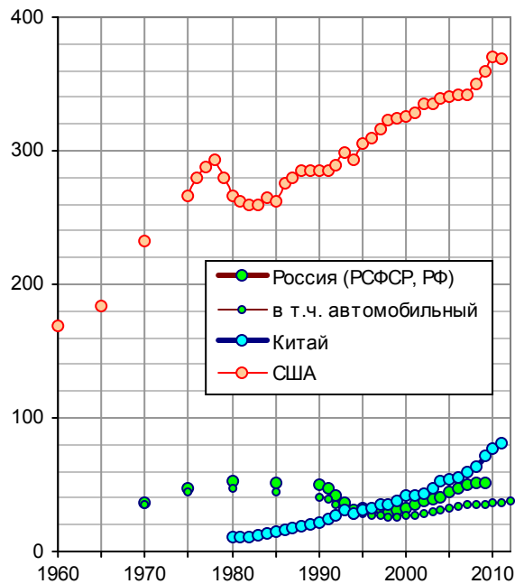
Производство автомобильного бензина, млн. тонн. Источники: [12, S.6, S.12]. Данные EIA в баррелях в день пересчитаны в тонны в год. Коэффициент пересчета принят для марки бензина "Regular", 1 баррель = 0,112 тонн.
